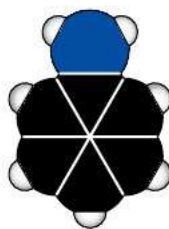
Рис. 75. Масштабная модель молекулы анилина
