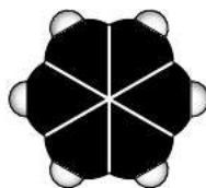
Рис. 25. Масштабная модель моле- кулы бензола
