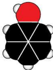
Рис. 42. Масштабная модель молекулы фенола
