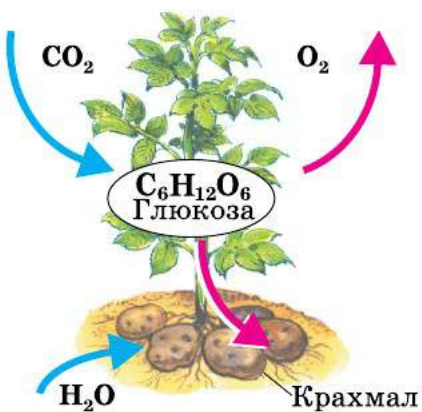
Рис. 1. Фотосинтез
