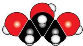
Рис. 40. Масштабная модель молекулы глицерина
