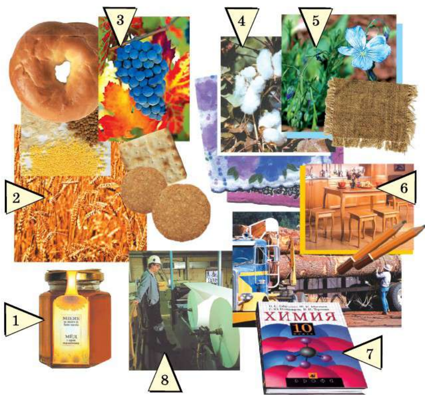
Рис. 65. Углеводы в жизни человека: 1—3 — продукты питания; 4, 5 — волокна и ткани (хлопчатобумажные 4, льняные 5); 6 — изделия из древесины; 7, 8 — бумага и изделия из неё
