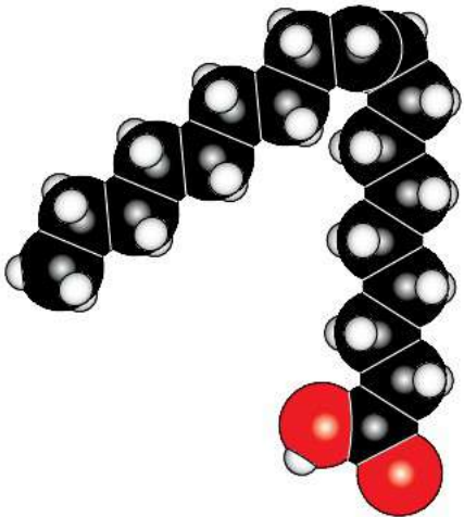
Рис. 50. Масштабная модель молекулы олеиновой кислоты
