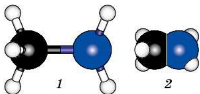
Рис. 74. Модель молекулы метиламина: 1 — шаростержневая; 2 — масштабная
