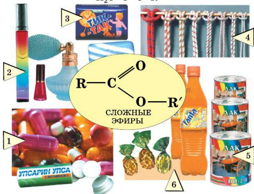
Рис. 58. Применение сложных эфиров: 1 — лекарственные средства; 2, 3 — парфюмерия и косметика; 4 — синтетические и искусственные волокна; 5 — лаки; 6 — производство напитков и кондитерских изделий
