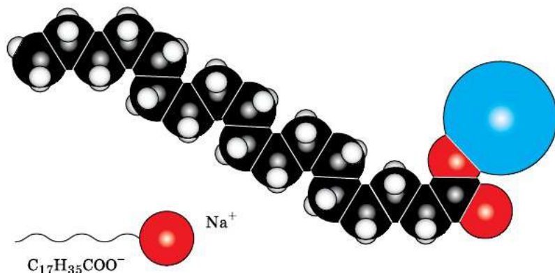
Рис. 61. Модель молекулы стеарата натрия в воде
