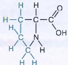
Пролин (про)
