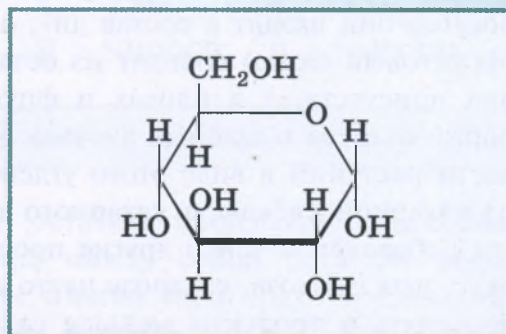
Рис. 25. Глюкоза
