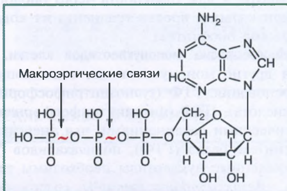
Рис. 42. АТФ
