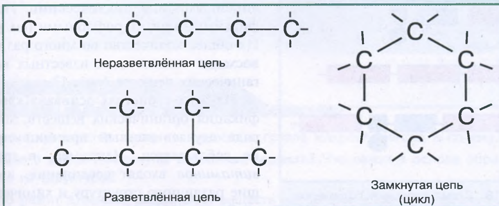
Рис. 16. Углеродный скелет
