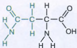
Аспарагин (асн)
