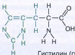
Гистидин (гис)*
