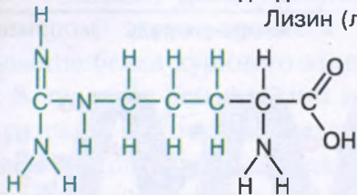
Аргинин (арг)*
