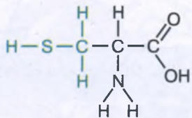
Цистеин (цис)
