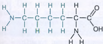
Лизин (лиз)
