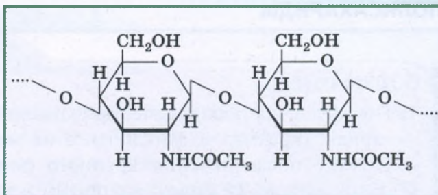
Рис. 29. Хитин
