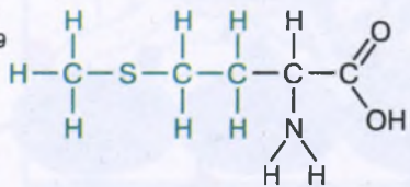
Метионин (мет)*
