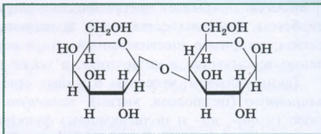
Рис. 28. Целлюлоза
